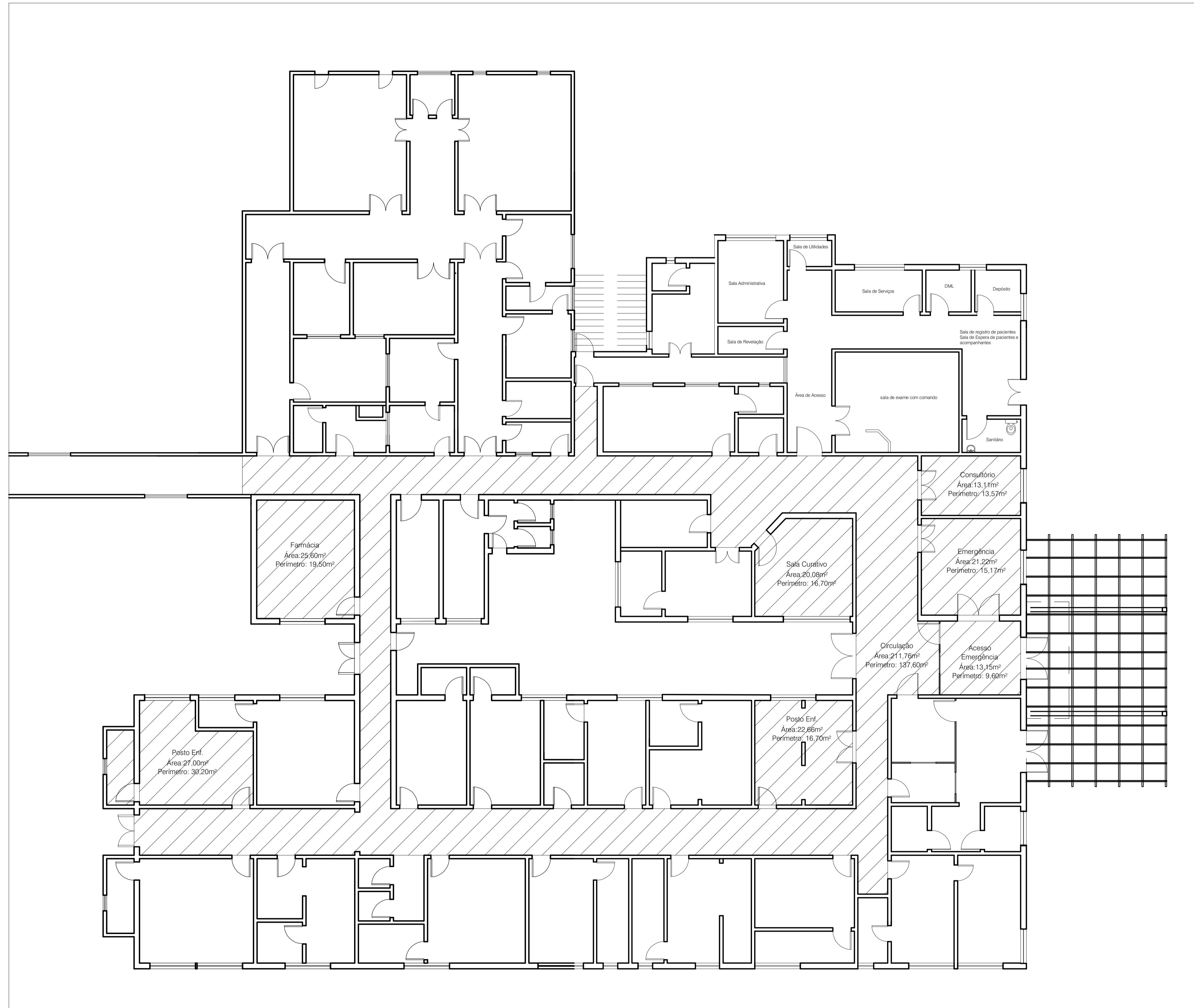
Planta Baixa ESC.: 1/100
