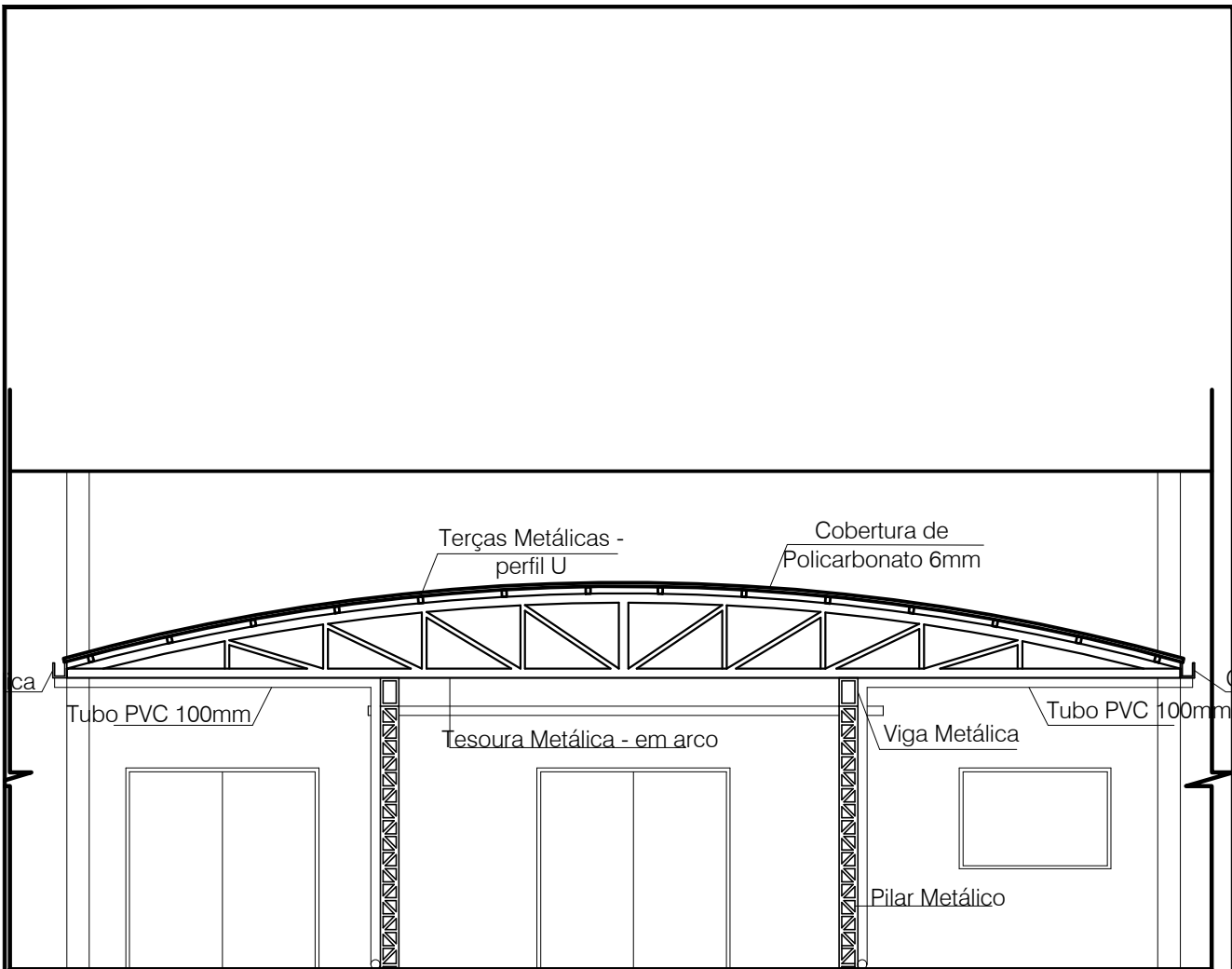
Fachada Frontal Esc.: 1/75
