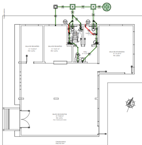
① Planta Baixa - Térreo Escala: 1/50
