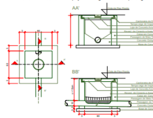
Detalhamento Caixa de Inspeção de Esgoto com Tampa Cega
