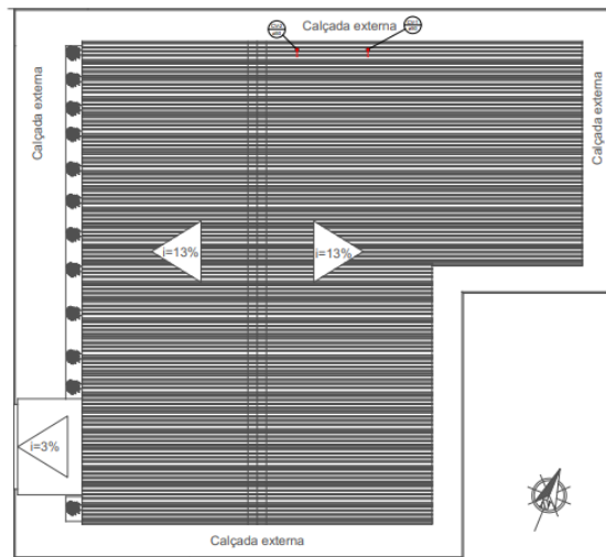
② Planta Baixa - Cobertura Escala: 1/50
