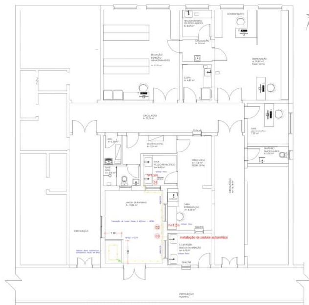
3 Planta Baixa Novo Layout CME Farmácia FHHTC ESCALA 1:50
